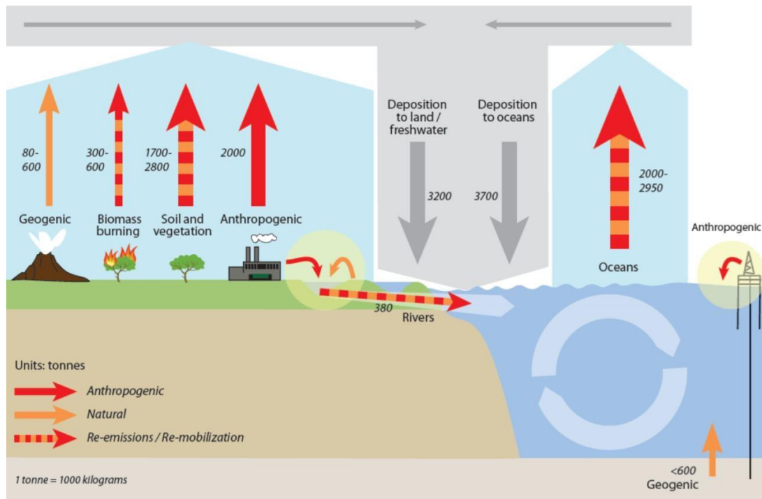
Figura 1. Ciclo biogeoquímico del mercurio (UNEP, 2013)
